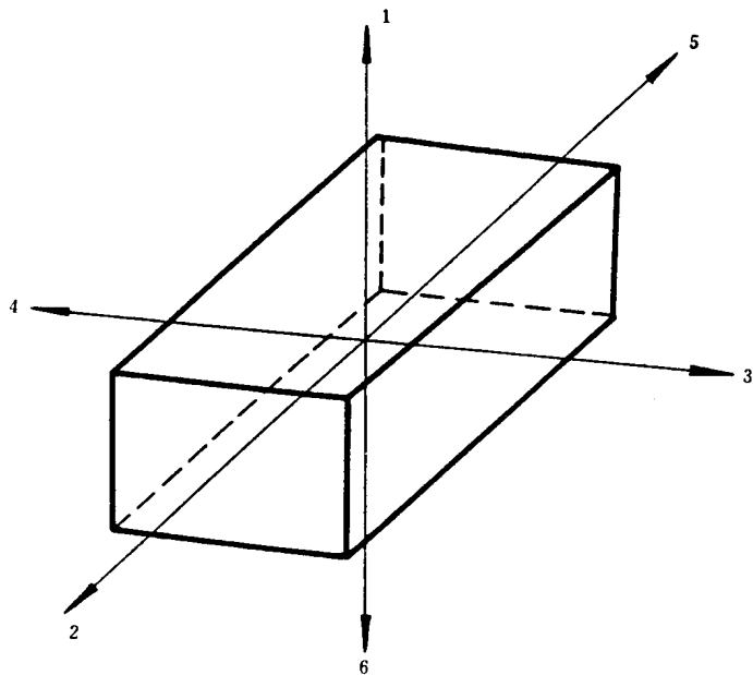
图 A4 矩形产品的主轴线 表 A1 矩形产品弹跳试验的方位和顺序
